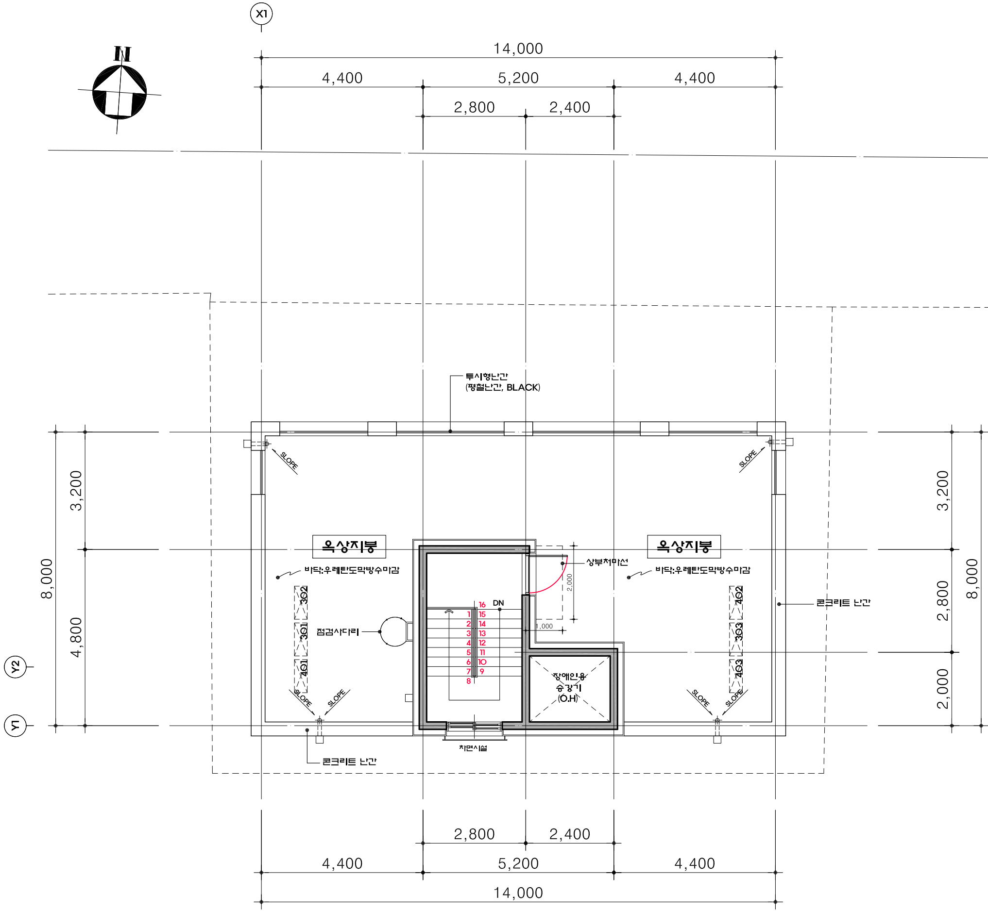
옥탑층 평면도 SCALE:1/100
