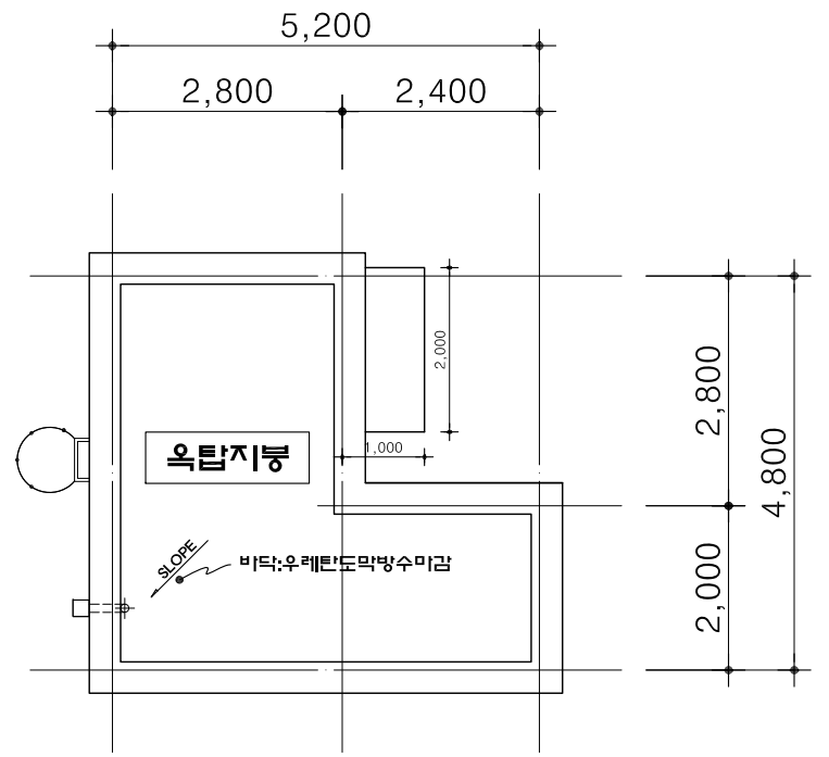
옥탑 지붕층 평면도 SCALE:1/100
