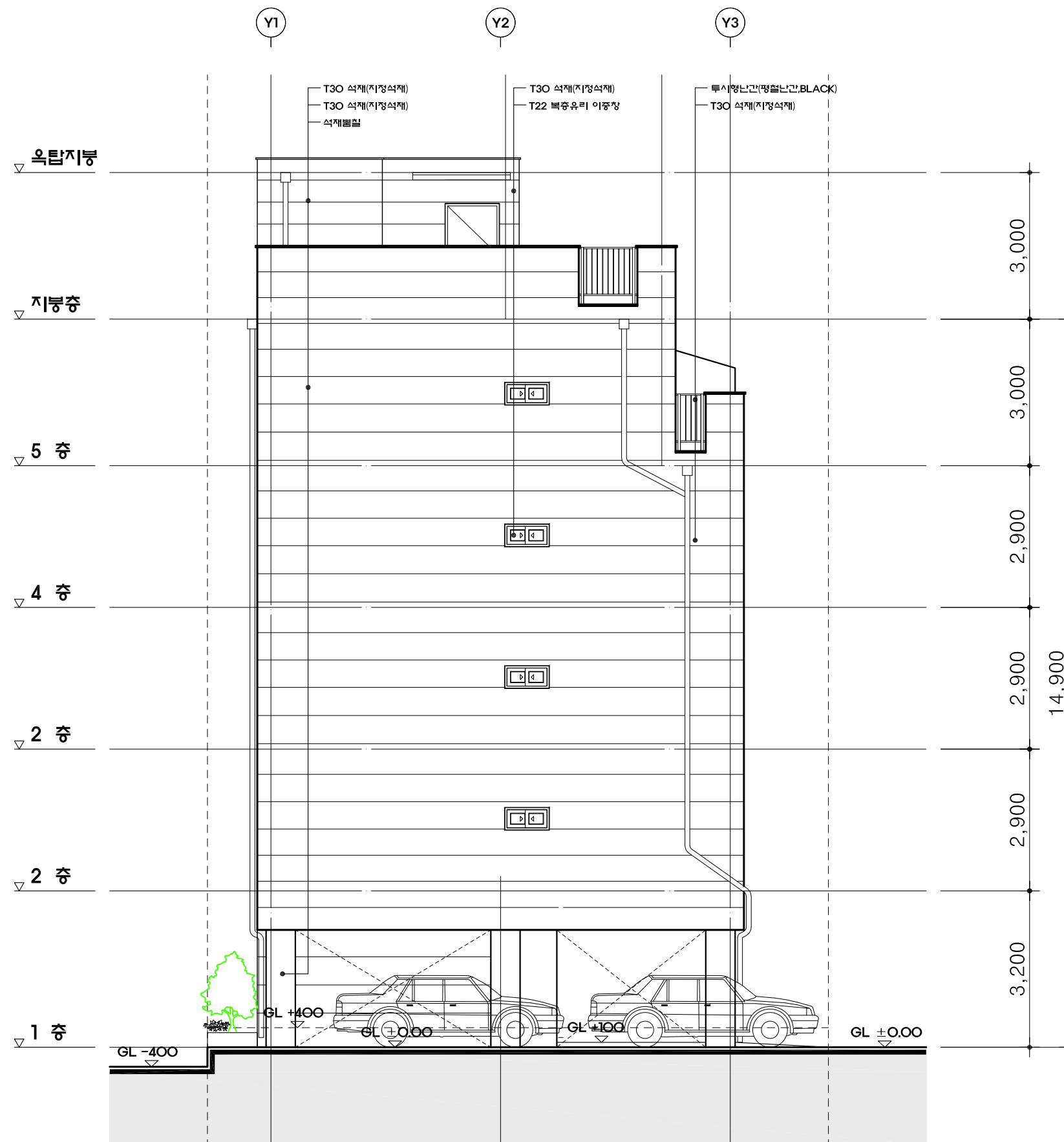
좌 측 면 도 SCALE:1/100
